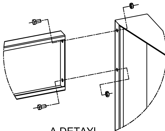
A DETAYI 2:1
